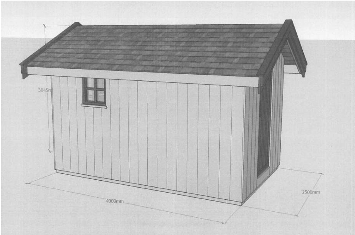
Målsatt tegning av uthuset
