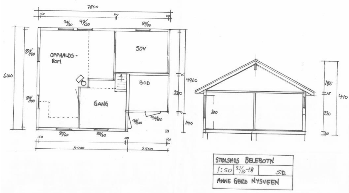
Figur 3. Rominndeling i omsøkt stølshus.
