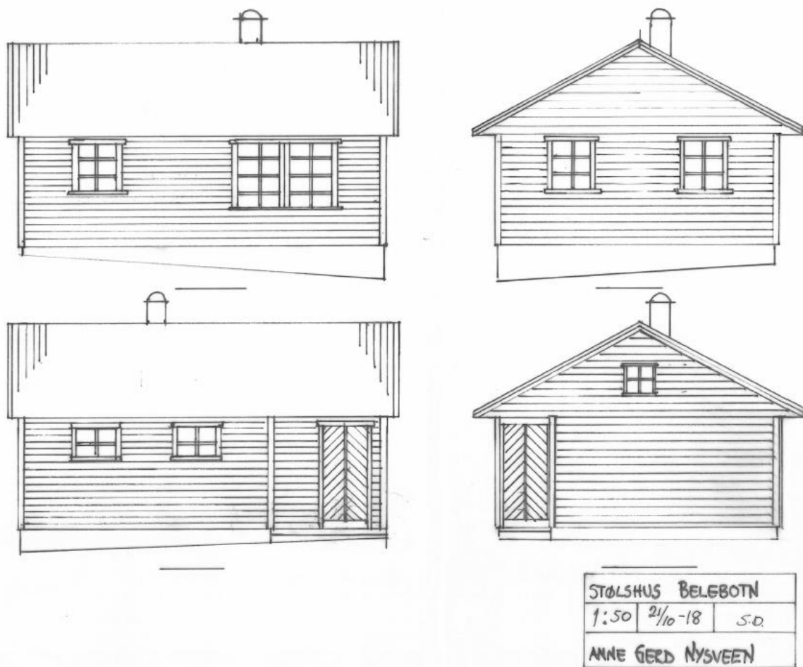
Figur 4. Teikningar frå byggesøknaden.
